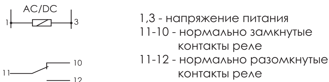
Рис.2 Назначение контактов.
