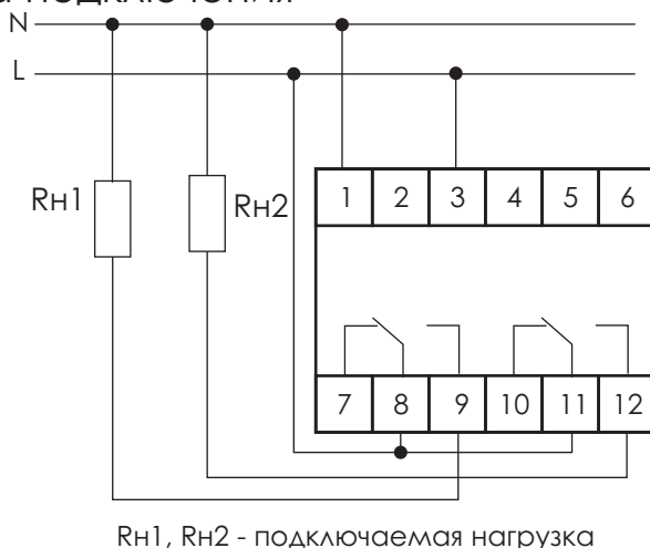
Рис.4 Схема подключения.
