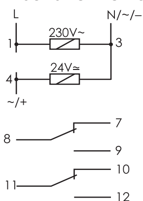
Рис.2 Назначение контактов.
