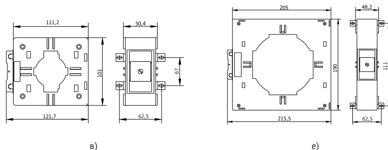
Рисунок 1. Габаритные и установочные размеры трансформаторов: а)ТТ-В30; б)ТТ-В40; в)ТТ-В60; г)ТТ-В80; д)ТТ-В100; е)ТТ-В120.
