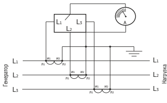
Рисунок 4. Схема подключения амперметра через трансформаторы тока
