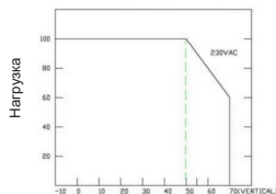
Кривая понижения в зависимости от окружающей температуры
